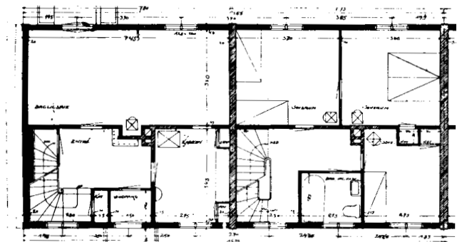
Tomannsbolig Plan 1:200
