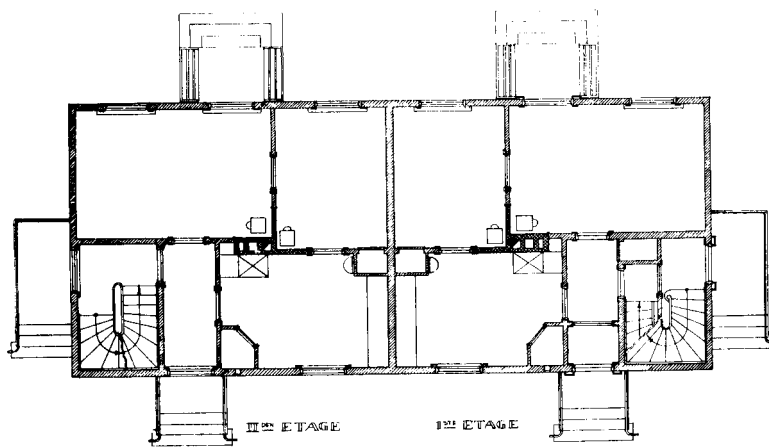
Firemannsbolig, 180 m 2 .
