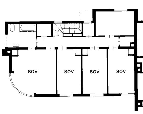
Heia II, 1. og 2. etasje 1:200
