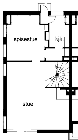
Planer Heia I, u., 1. og 2. etasje 1:200
