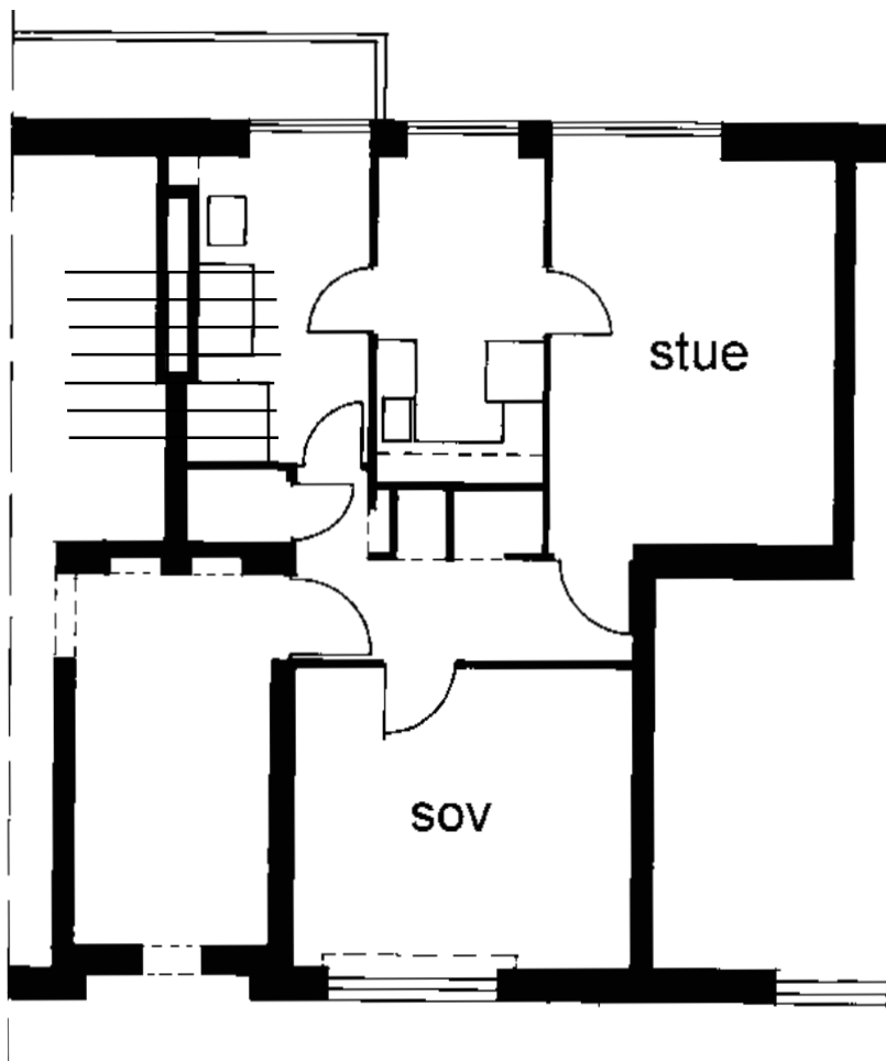
Leilighetsplan 1:100
